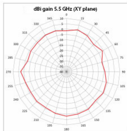
5 GHz Antenna
